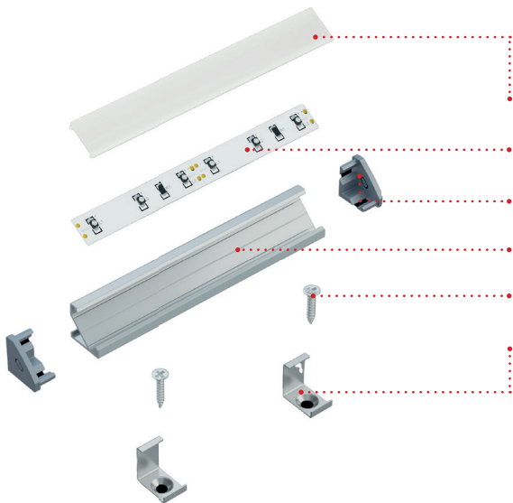
Axonometric projection before assembly using mounting clips and screws Rzut aksonometryczny przed montażem z wykorzystaniem uchwytów oraz wkrętów
