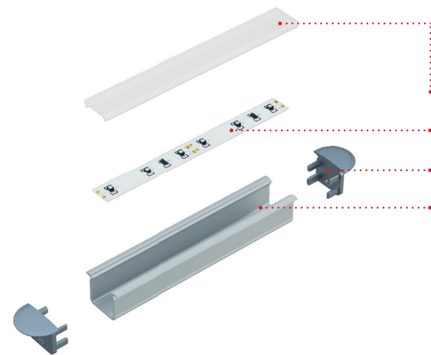
Axonometric projection before assembly Rzut aksonometryczny przed montażem
