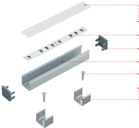
Axonometric projection before assembly using mounting clips and screws Rzut aksonometryczny przed montażem z wykorzystaniem uchwyty oraz wkrętów
