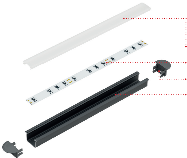
Axonometric projection before assembly Rzut aksonometryczny przed montażem
