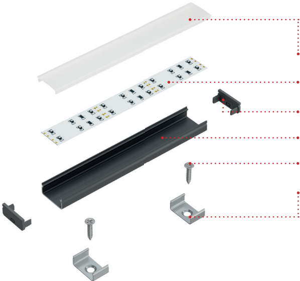
Axonometric projection before assembly using mounting clips and screws Rzut aksonometryczny przed montażem z wykorzystaniem uchwyty oraz wkrętów
