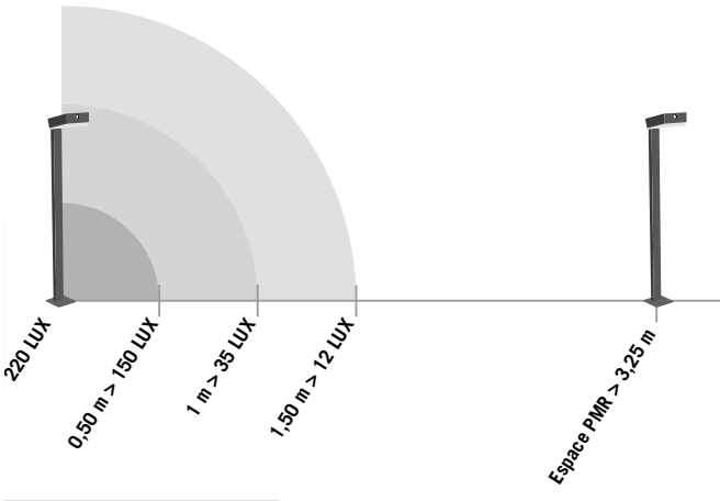
IMPLANTATION LUX /DISTANCE TEST RÉALISÉ AVEC UNE BORNE TD07K106 500 LM
