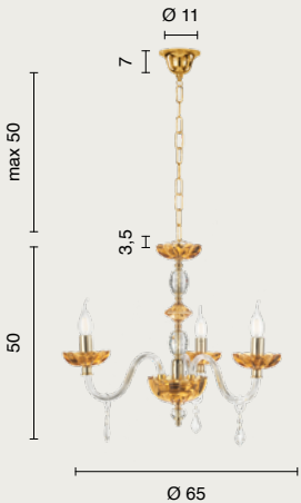
lampadario chandelier LP.PATRICIA/3A METEL: OLP0199
