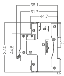
DPN
