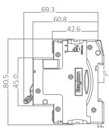
MCB-1P
