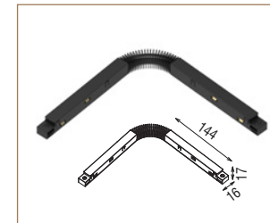
48V-Q1/Q2 FLEXIBLE CONNECTOR
