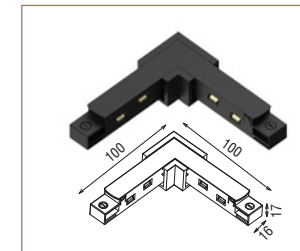
48V-Q1 CONNECTOR MINI
